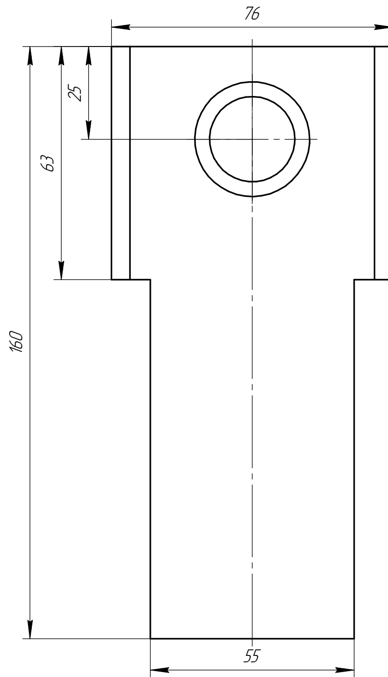
Дет. поз. 4 (1:1)
