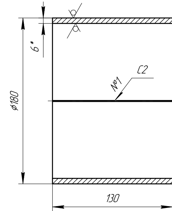
Дет. поз. 6
