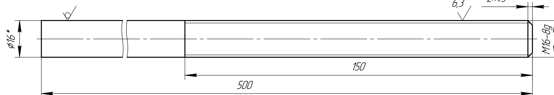
Дет. поз. 5 (1:1)
