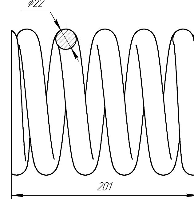
Дет. поз. 6
